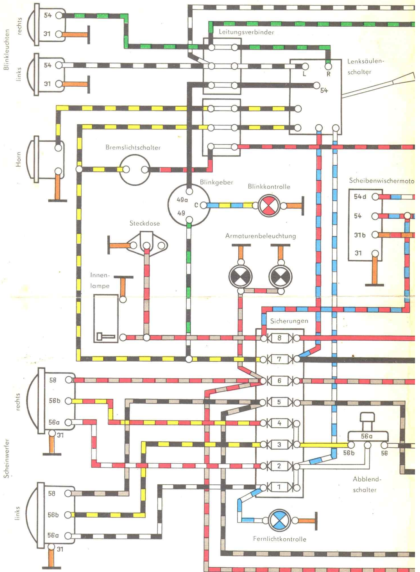
Trabant 600 / 601
